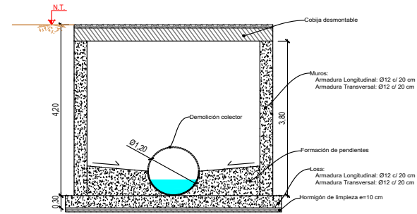
SECCIÓN A-A
