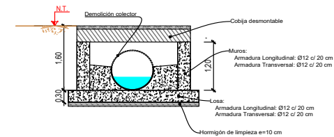
SECCIÓN A-A
