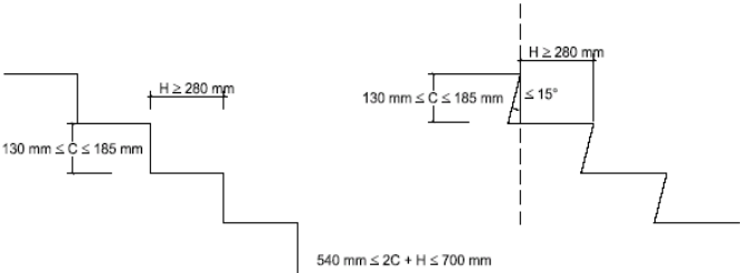
Figura 4.2 Configuración de los peldaños.
