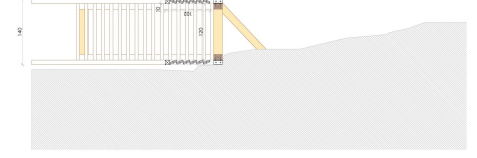
SECCION PLANTA ESCUELA PARA EL BARRIO - ESCUELA T29 (CORTA)
