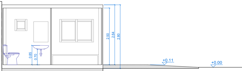
Sección transversal A-A'
