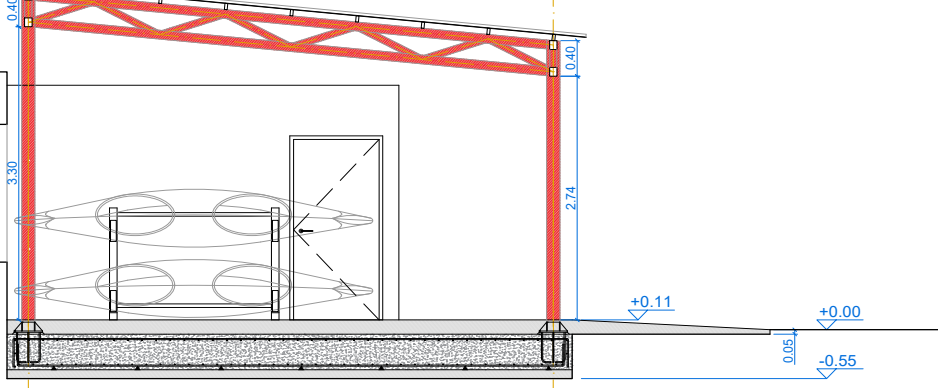
Sección transversal B-B'
